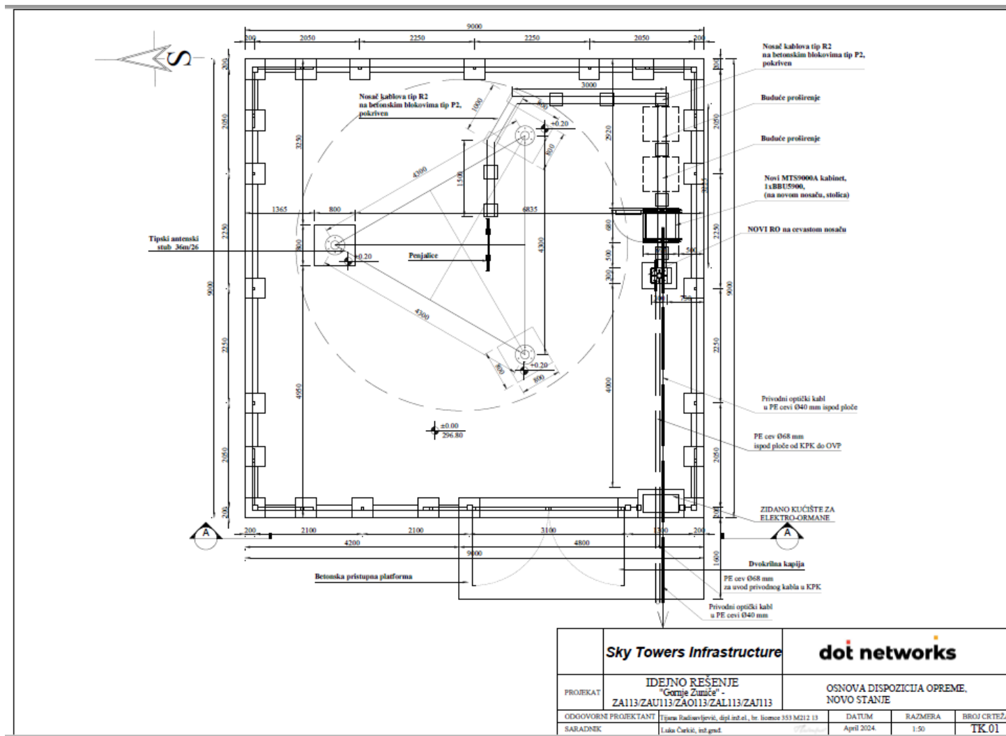
Slika 3.2.2 Osnova dispozicije opreme – novo stanje
