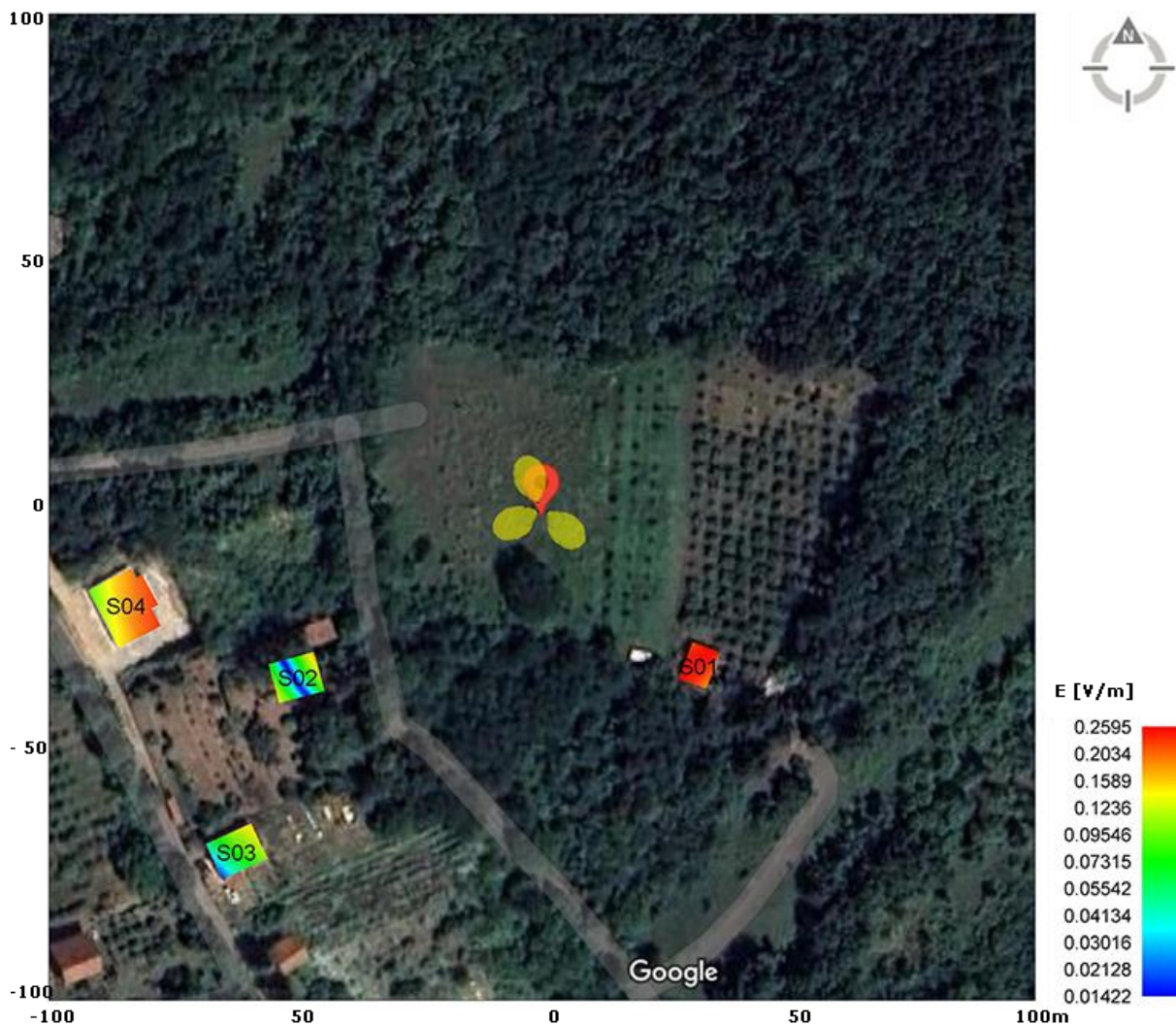
Slika 6.7. Rezultati proračuna jačine električnog polja u objektima kada sistem GSM900 operatera Telekom Srbija radi maksimalnim kapacitetom
